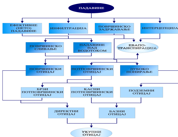
Слика 3 - Шематски приказ генезе укупног отицаја (Николић, Ј., 2004) Figure 3 - Schematic illustration of the total runoff genesis
